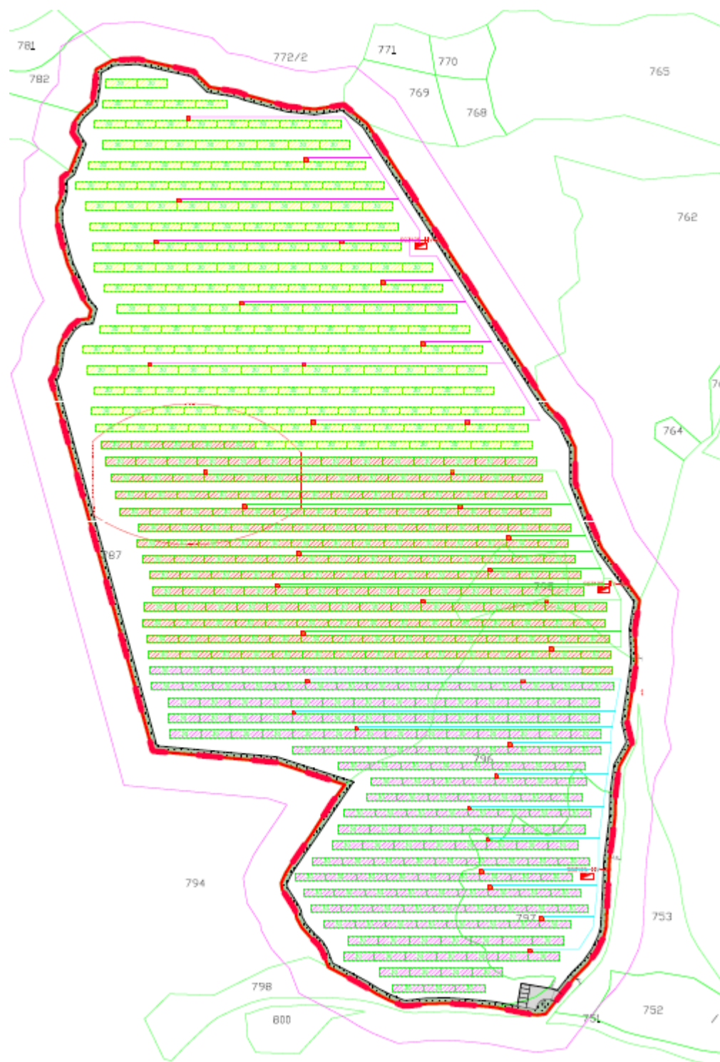
3.4 Распоред на стринговите по трафостаници
