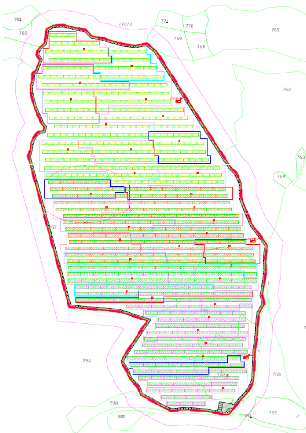
3.3 Распоряд на стринговите по DC собирни кутии
