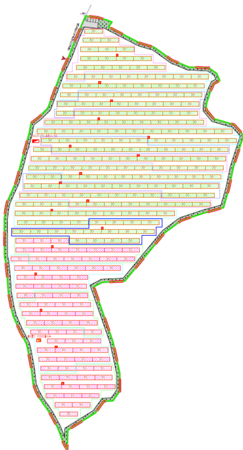
3.3 Распоред на стринговите по DC собирни кутии
