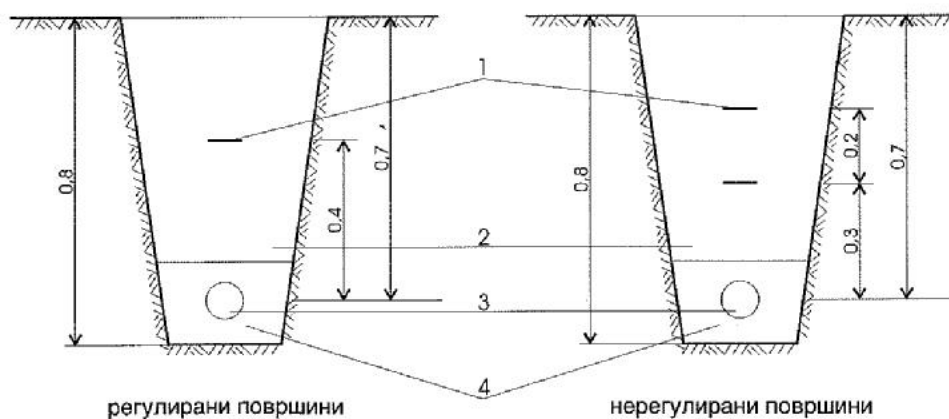
Слика 2-16. Полагање на НН кабел на рагулирани и нерегулирани површини
