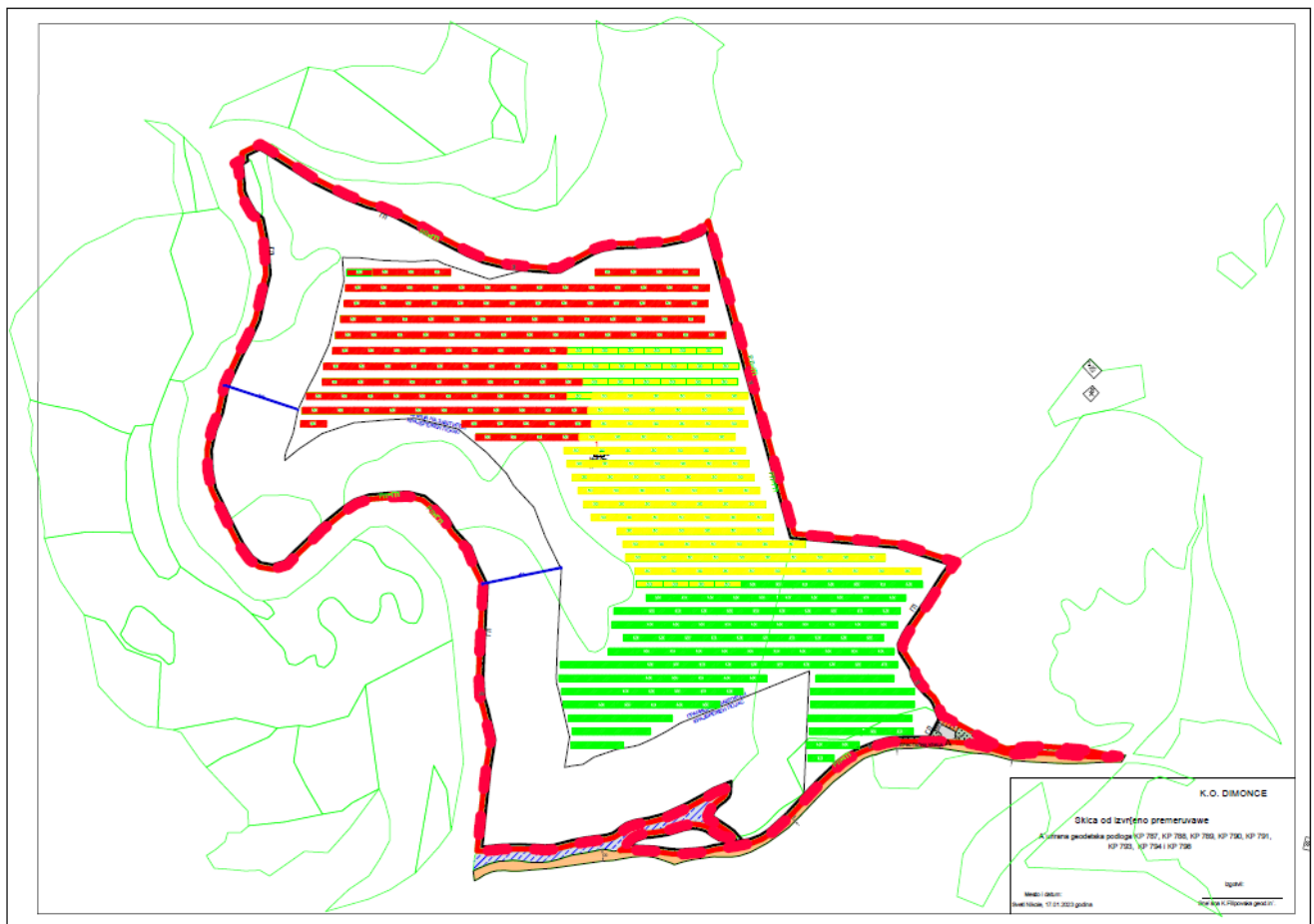
3.4 Распоред на стринговите по трафостаници
