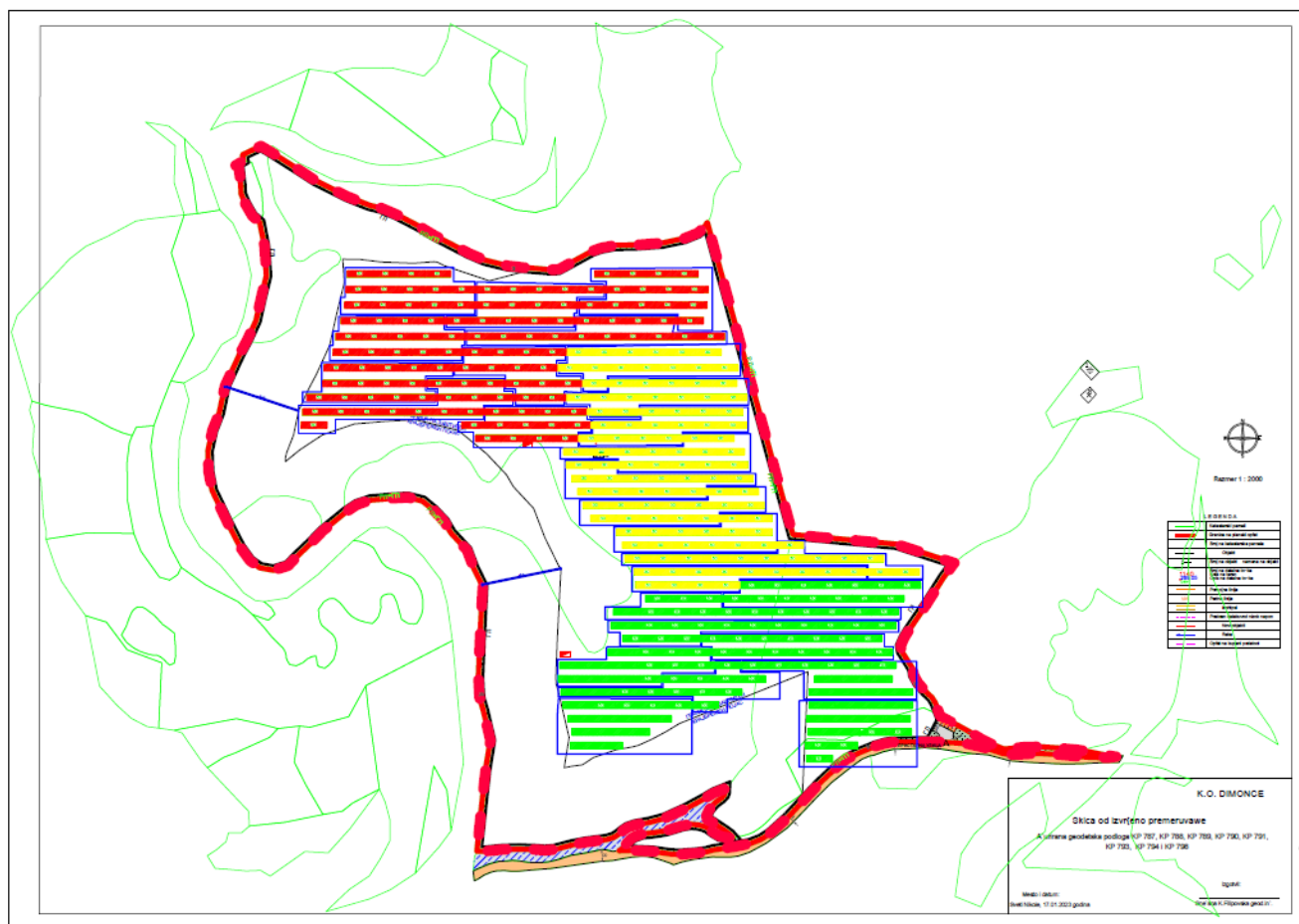
3.3 Распоред на стринговите по DC собирни кутии
