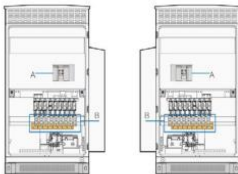
Слика 2-10 Ормар за DC развод – Распоред на опрема
