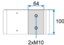
Слика 2-14 детал (плочка) за заземјување на ИТС
