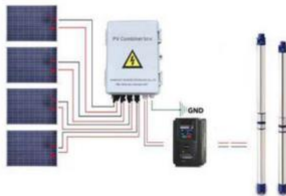
Слика 2-7 Принцип на работа на DC собирна кутија
