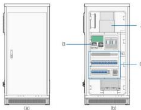
Слика 2-11 Ормар за контрола и управување
