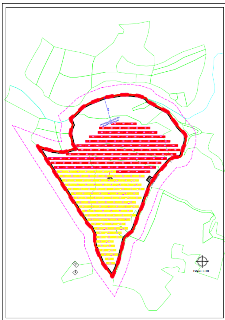
3.4 Распоред на стринговете по трафостаници
