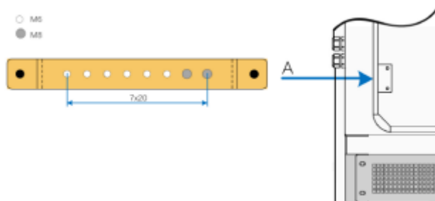
Слика 2-12 Шина за изедначување на потенцијал
