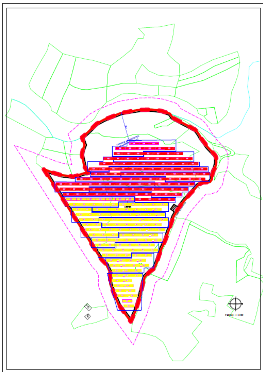
3.3 Распоряд на стринговите по DC собирни кутии
