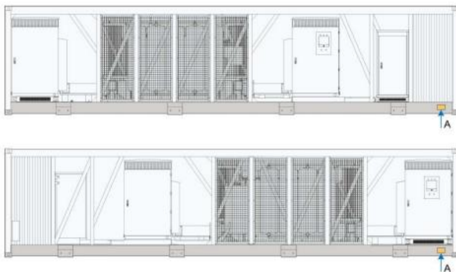
Слика 2-13 Места за заземјување на ИТС
