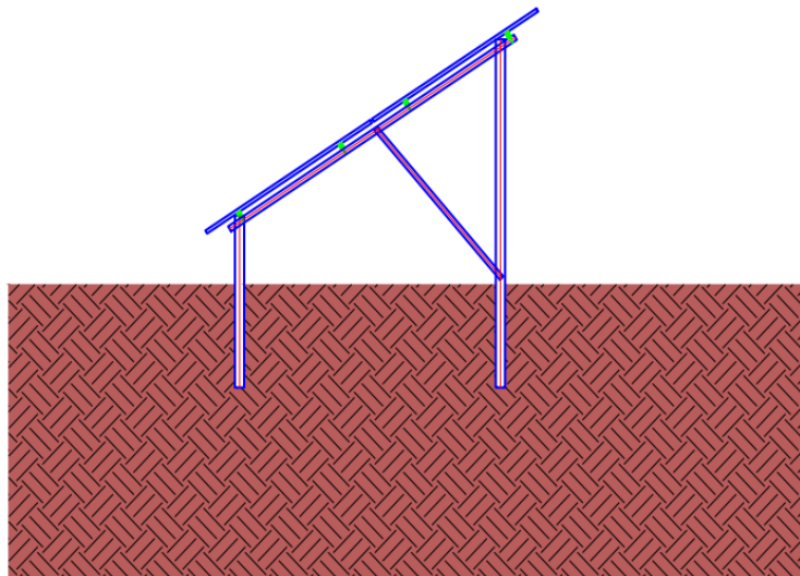
Слика 2-5 Конструкција за ФН панели
