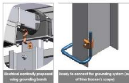
Слика 2-15 детал за заземјување на металната конструкција на панели
